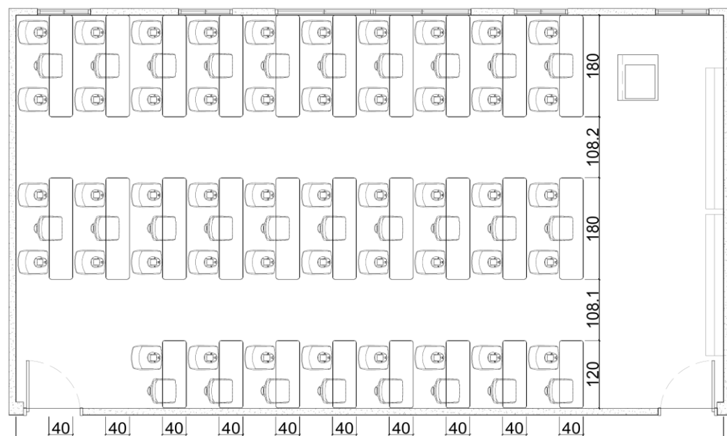
知武 207 · 規劃配置
