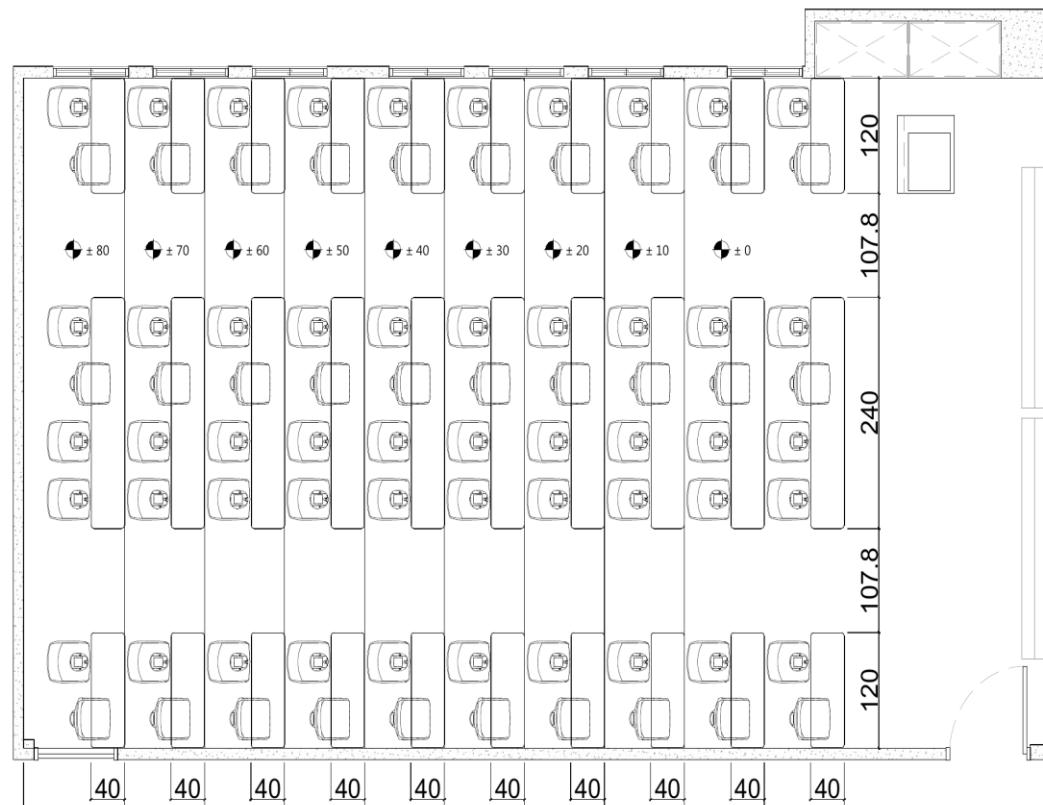
知武 209・新教室規劃配置圖
