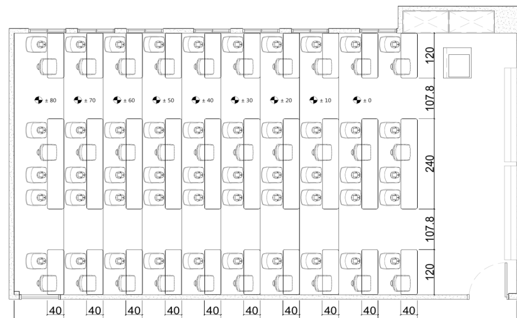
知武 209 · 規劃配置
